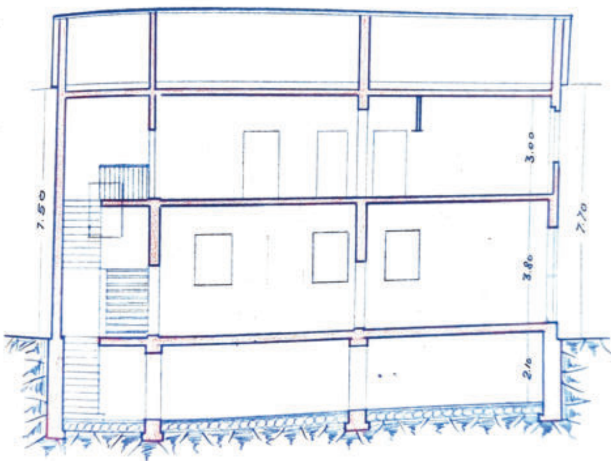
SEZIONE A-B-
