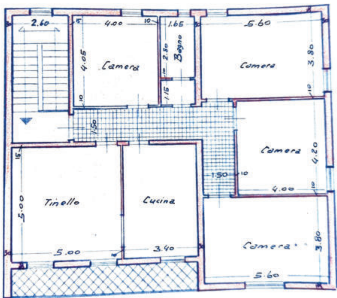
PIANO PRIMO
