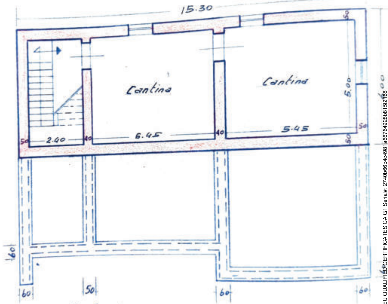
Pianta fondazioni e scantinato
